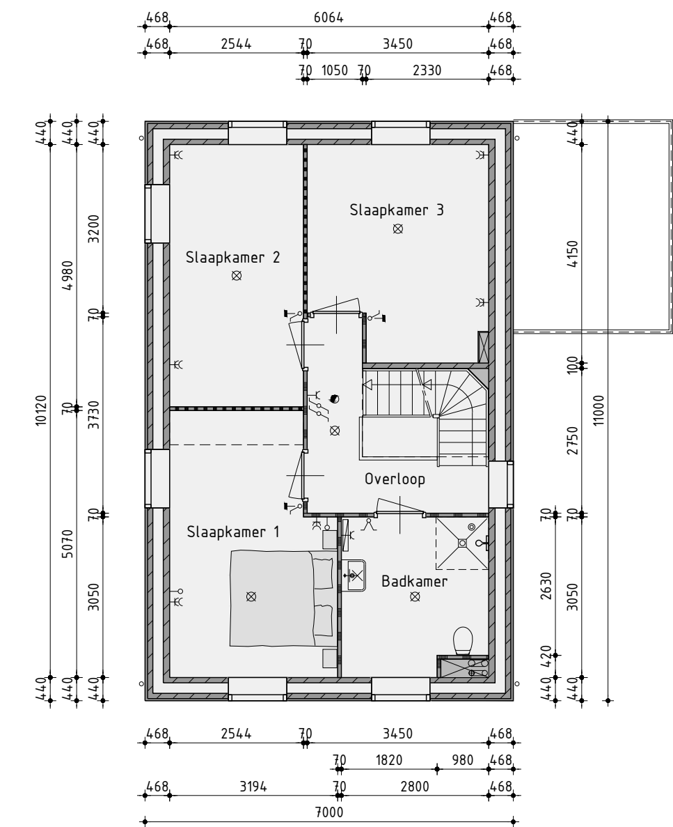
1ste Verdieping
