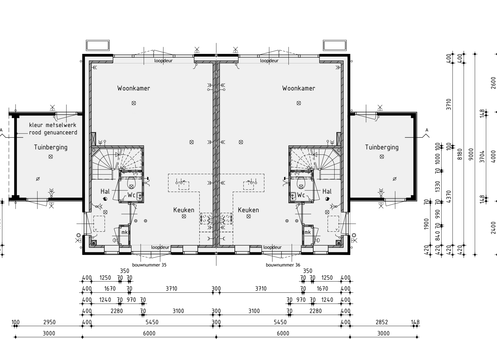
Begane grond
