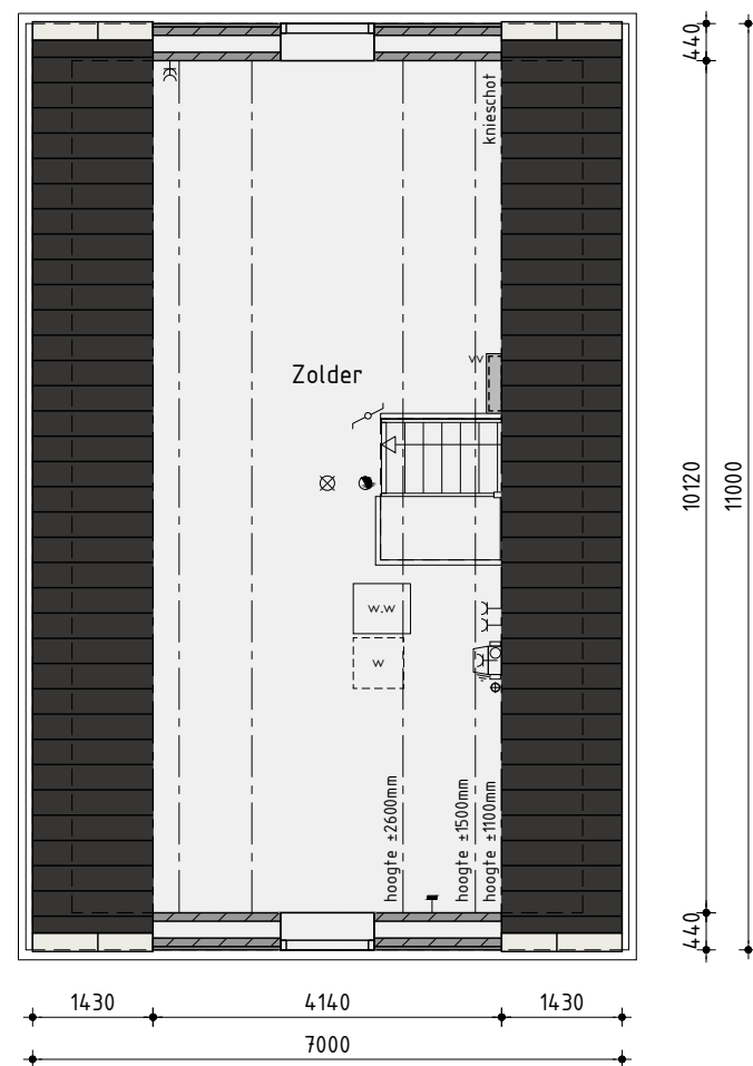
2de Verdieping
