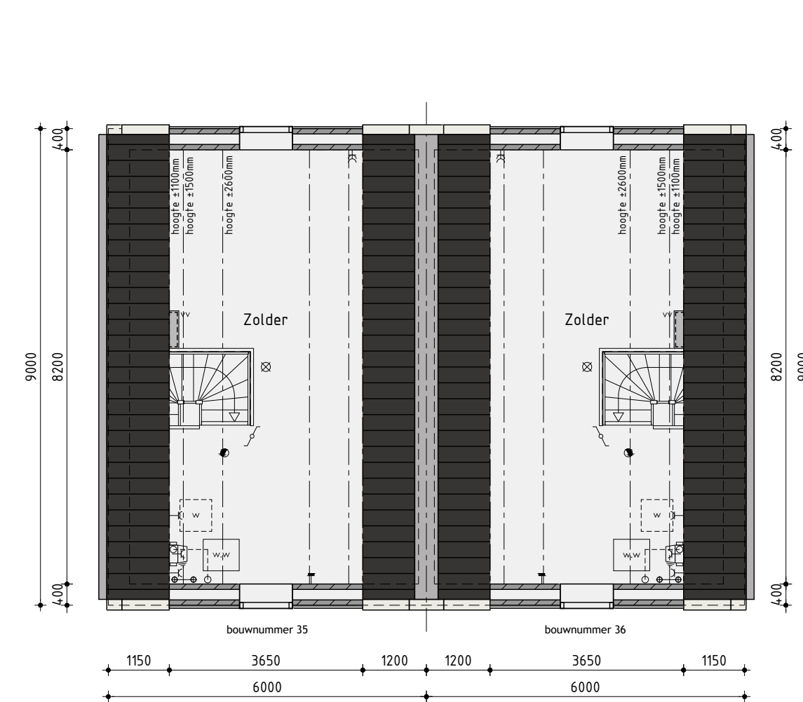
2de Verdieping
