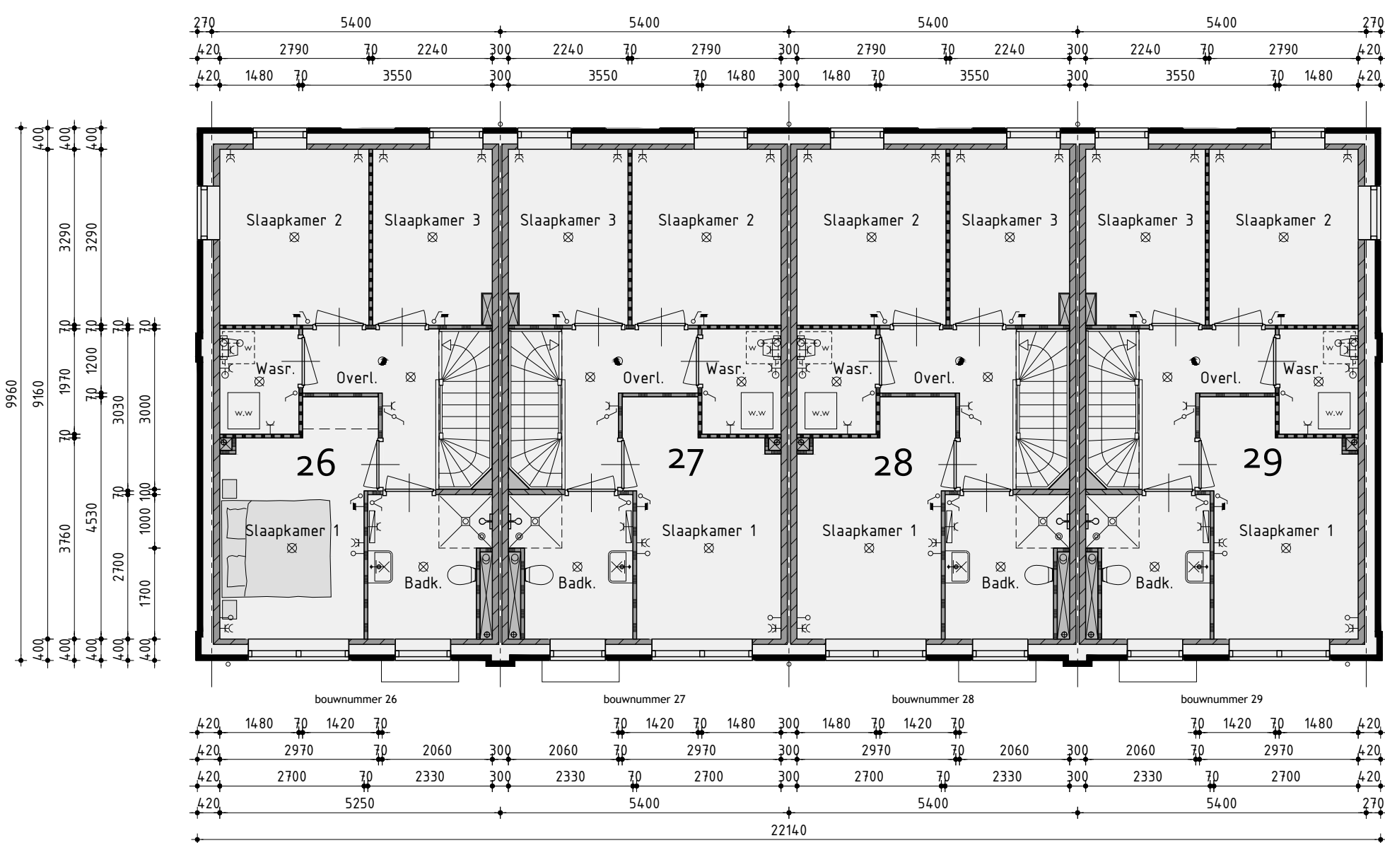
1ste verdieping
