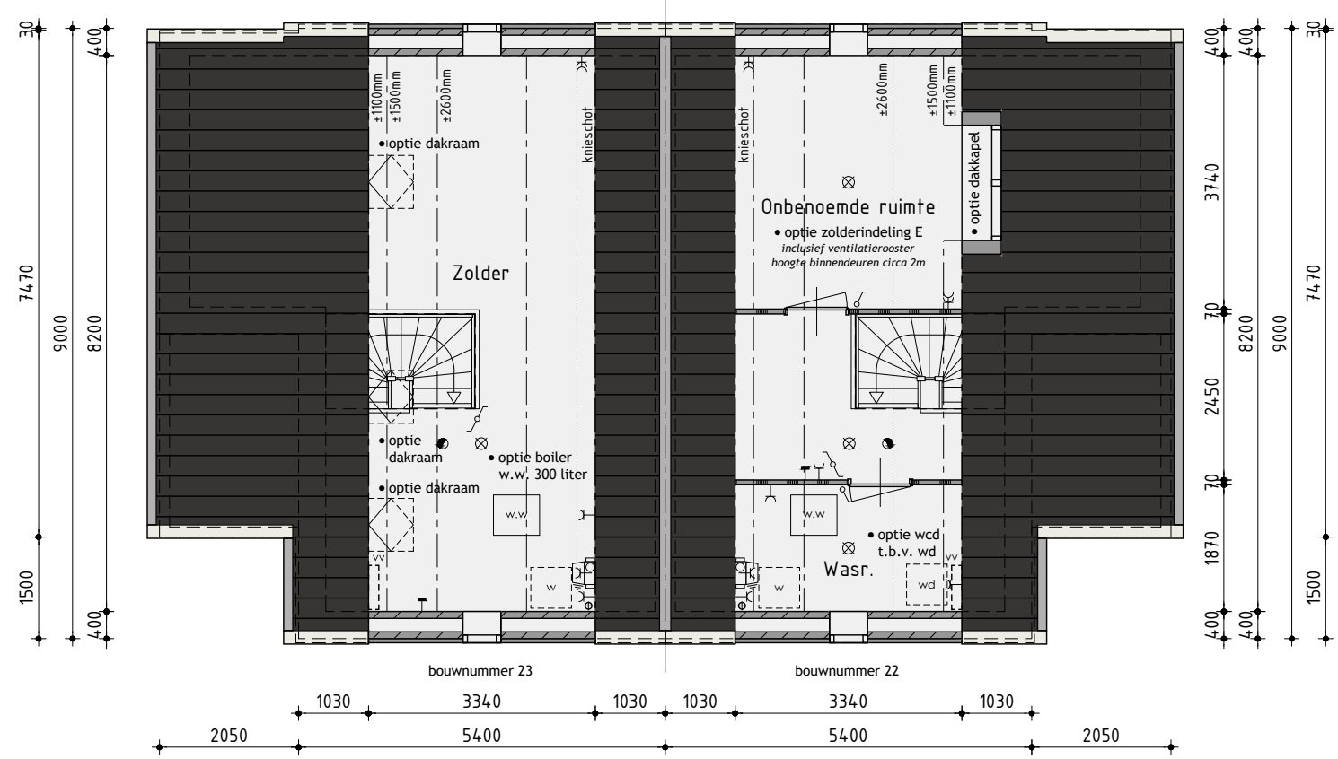
2de Verdieping
