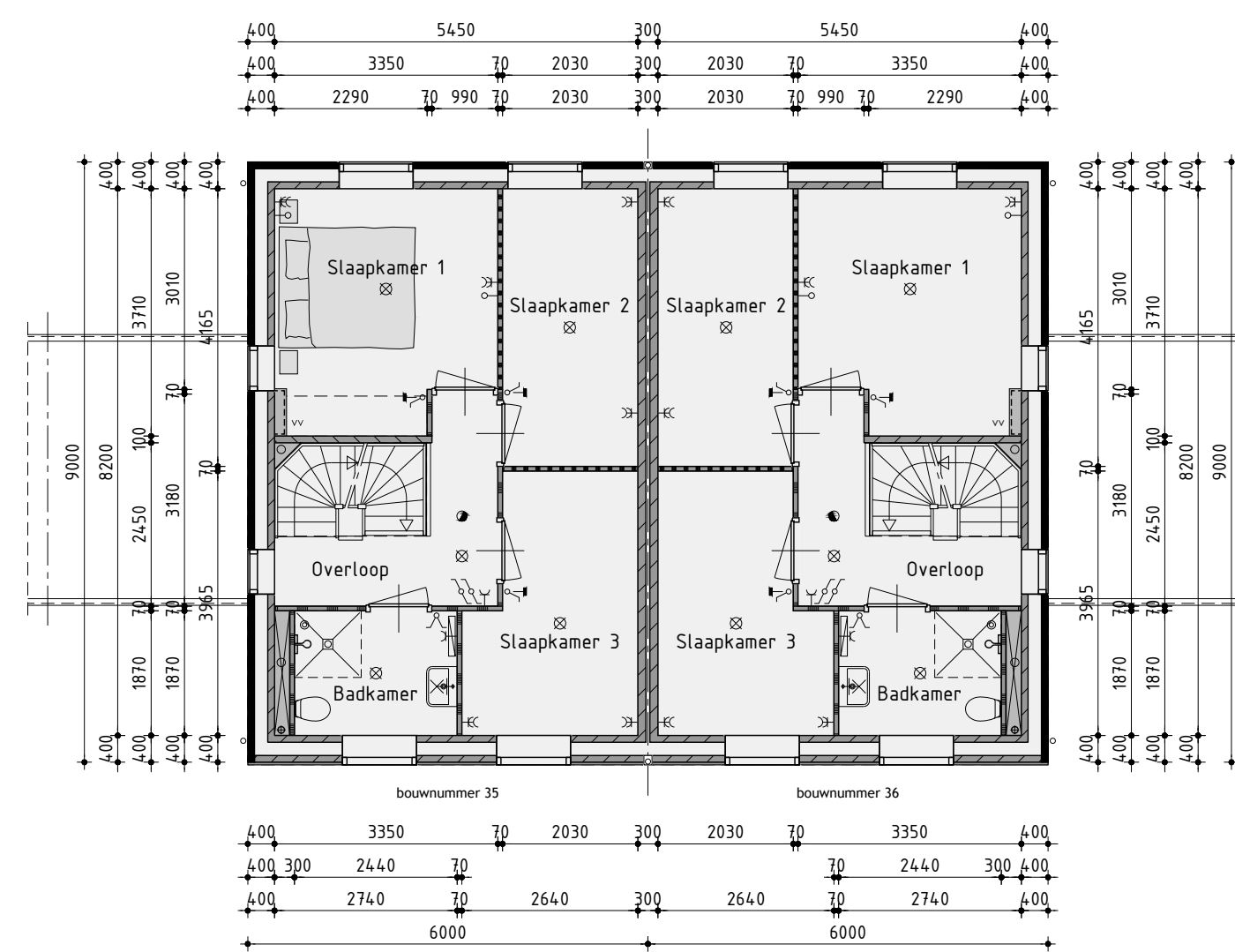
1ste Verdieping
