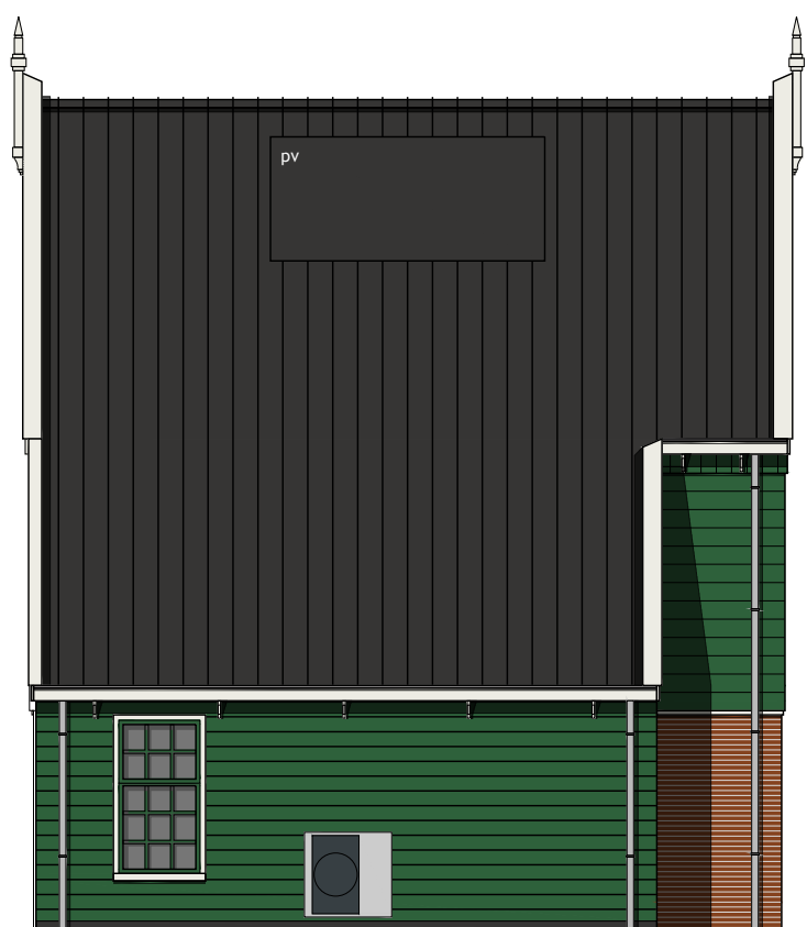
Linker zijgevel
