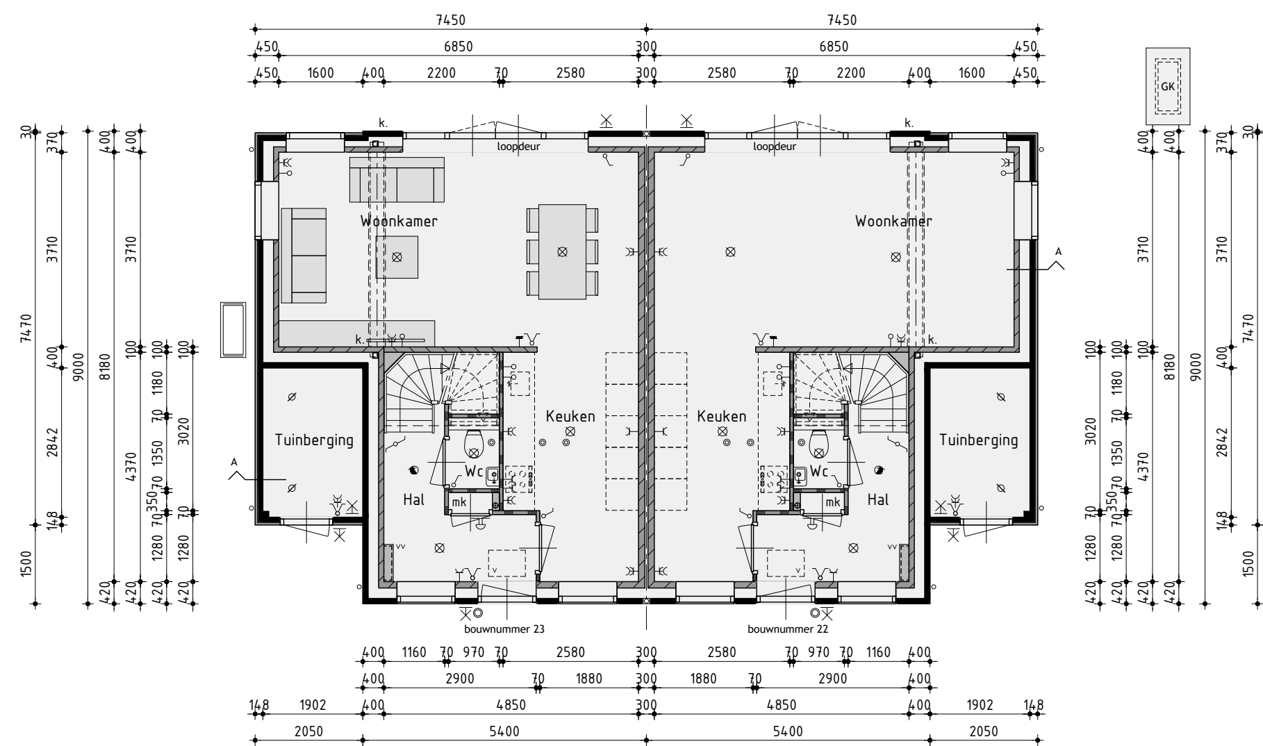
Begane grond
