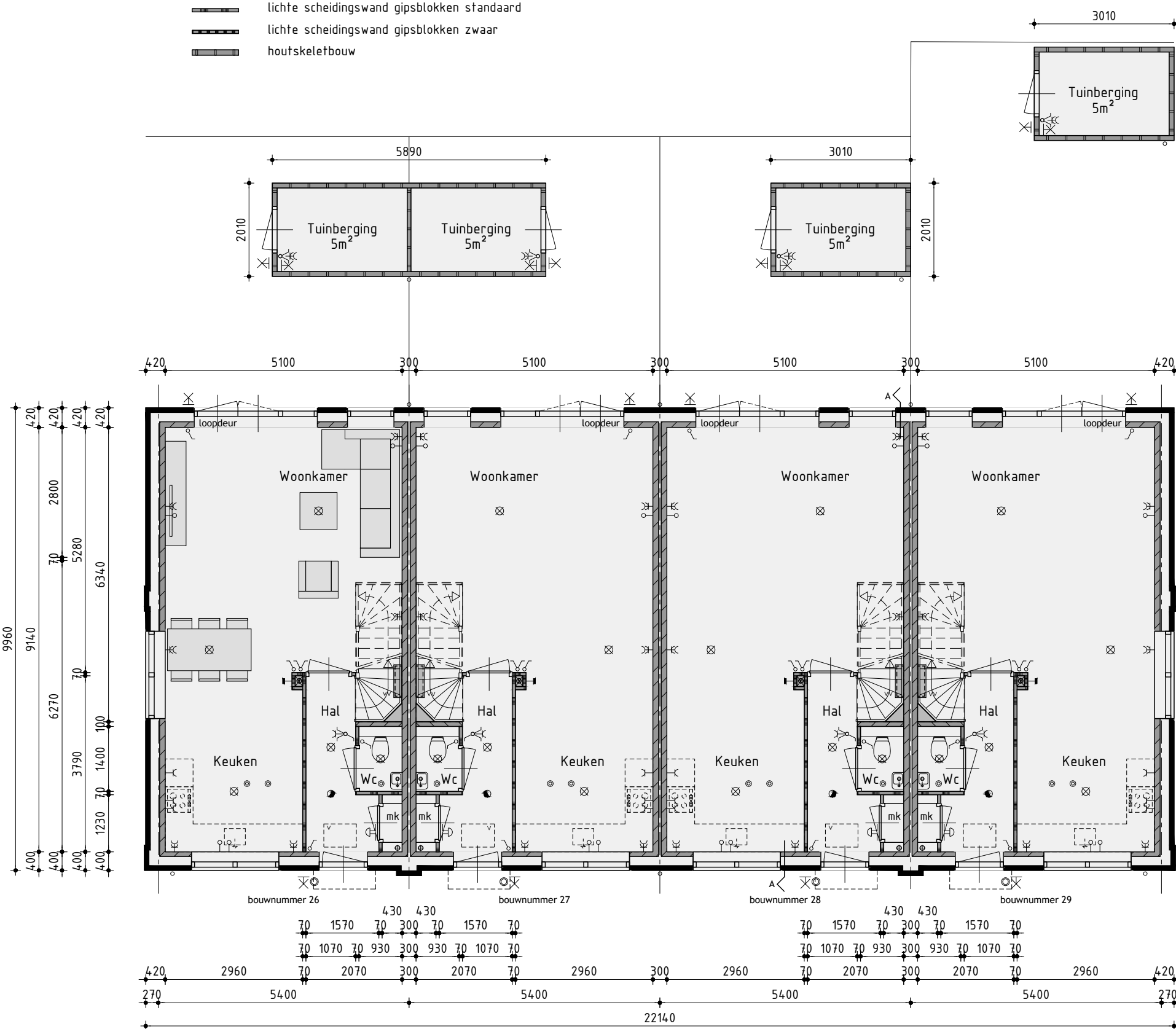
Begane grond
