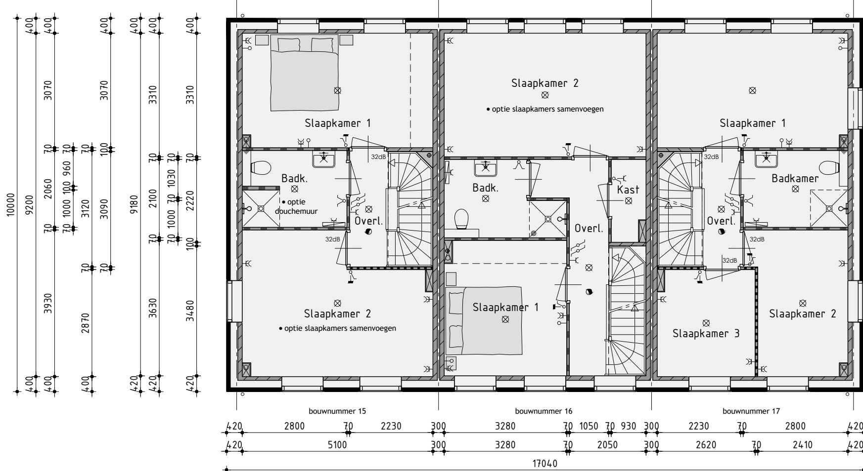
1ste Verdieping
