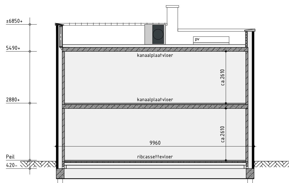
Principe doorsnede A-A
