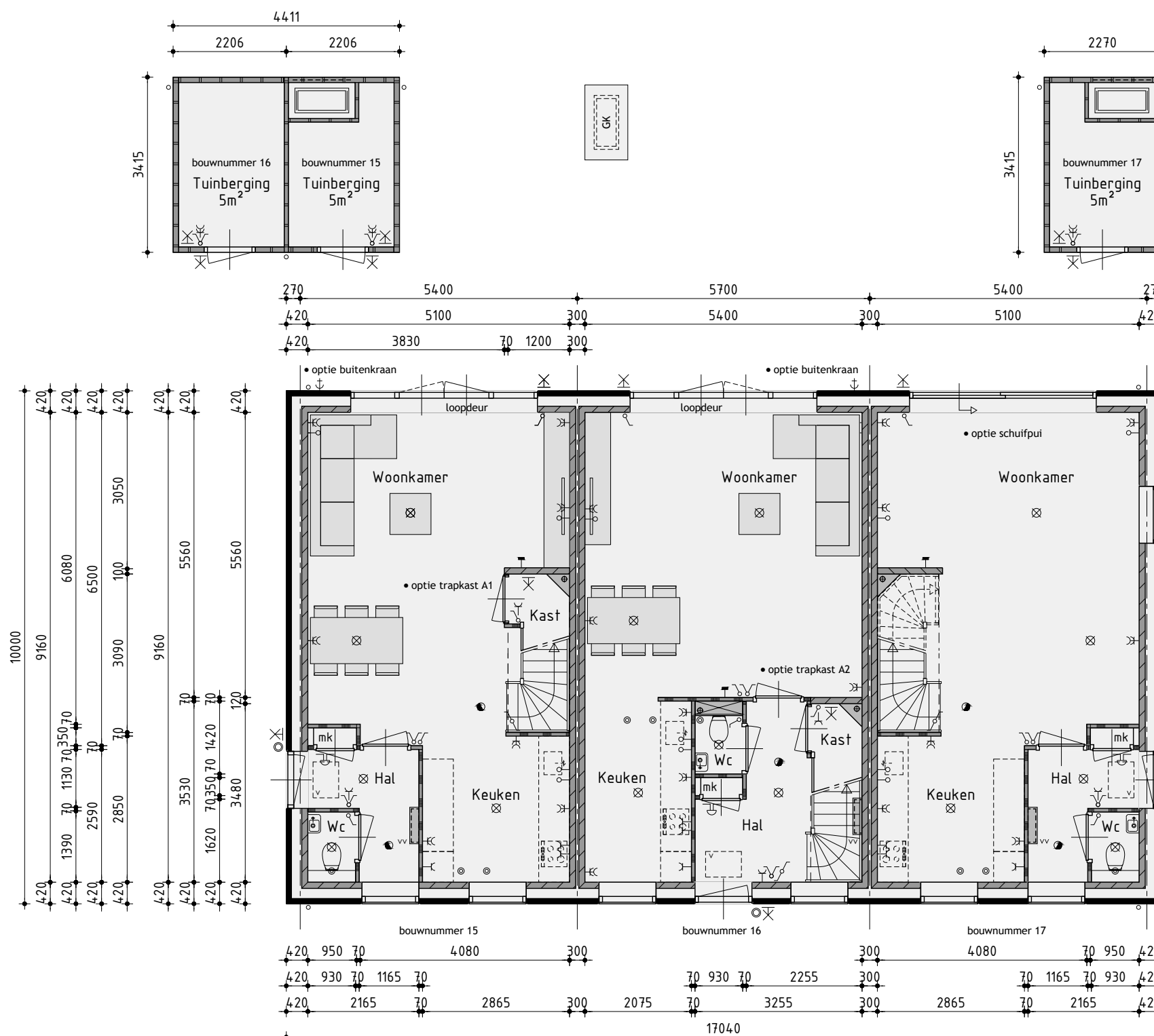
Begane grond
