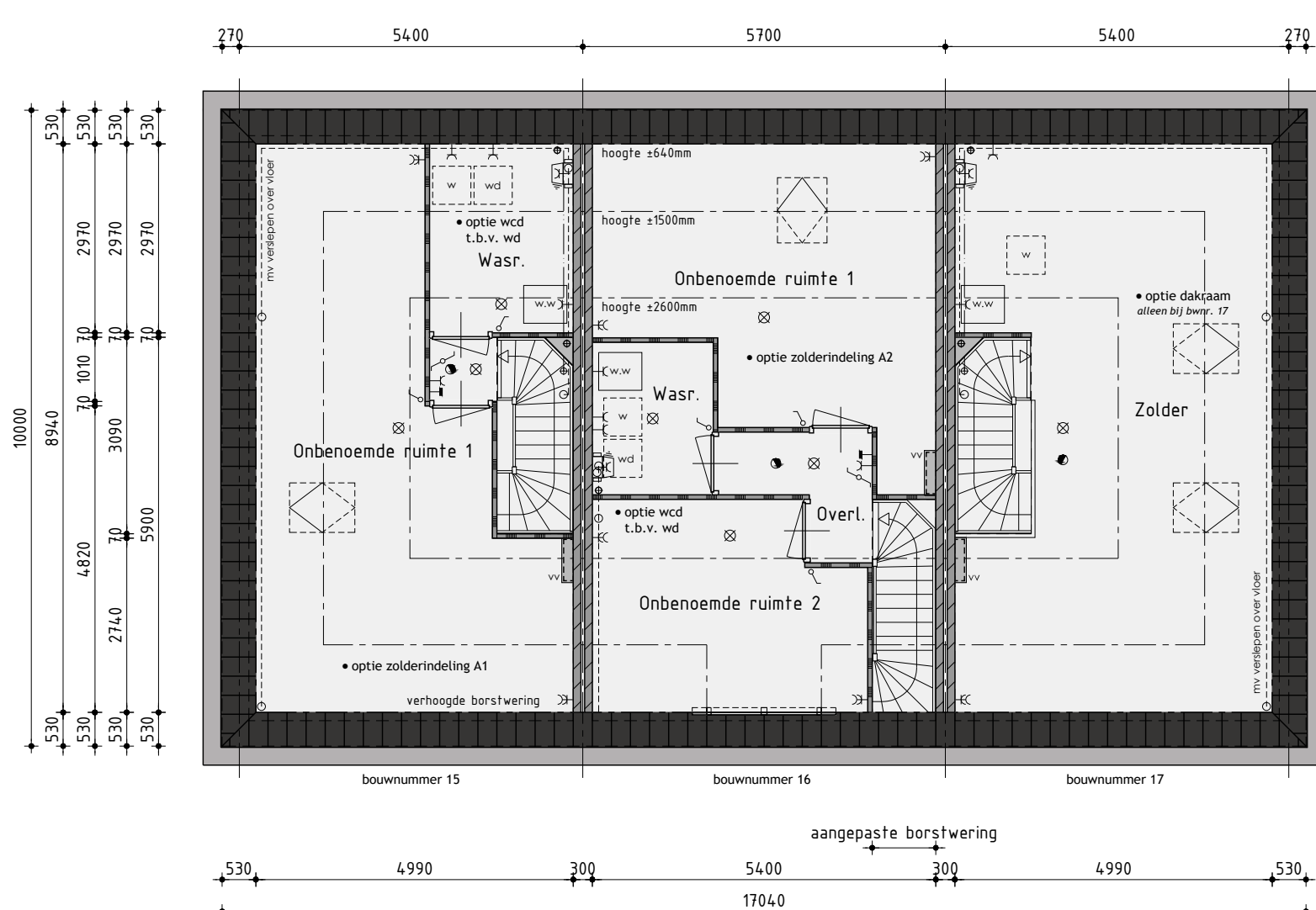
2de Verdieping
