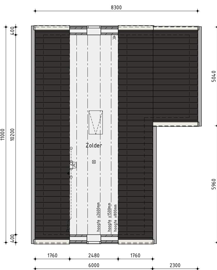
2de Verdieping
