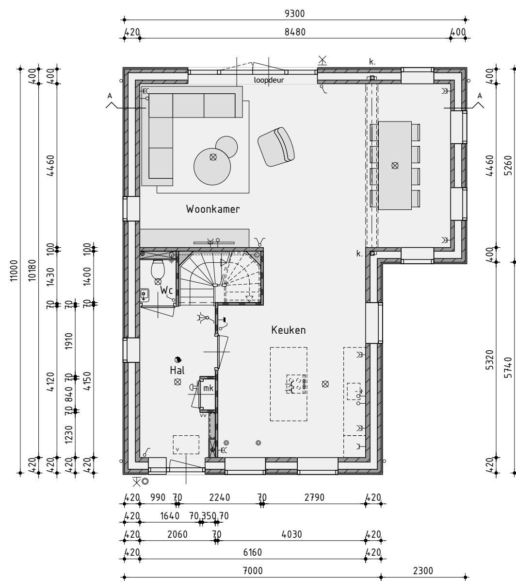
Begane grond
