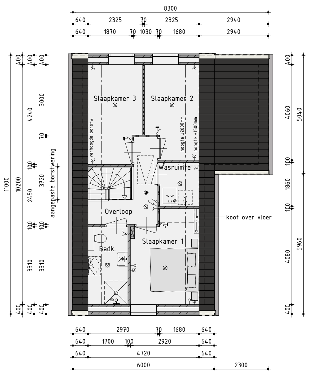
1ste Verdieping
