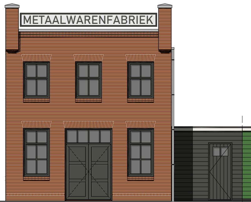
Voorgevel
