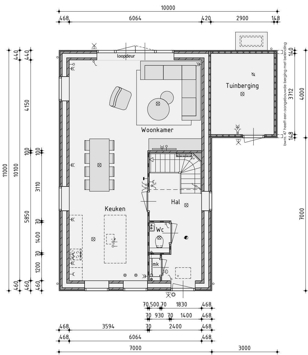
Begane grond
