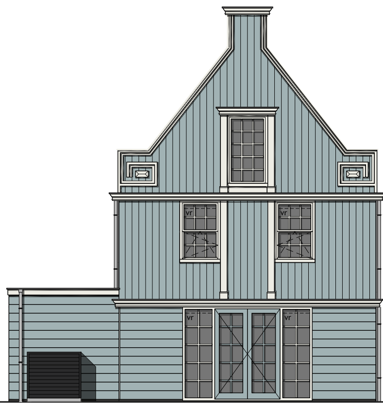
Achtergevel
