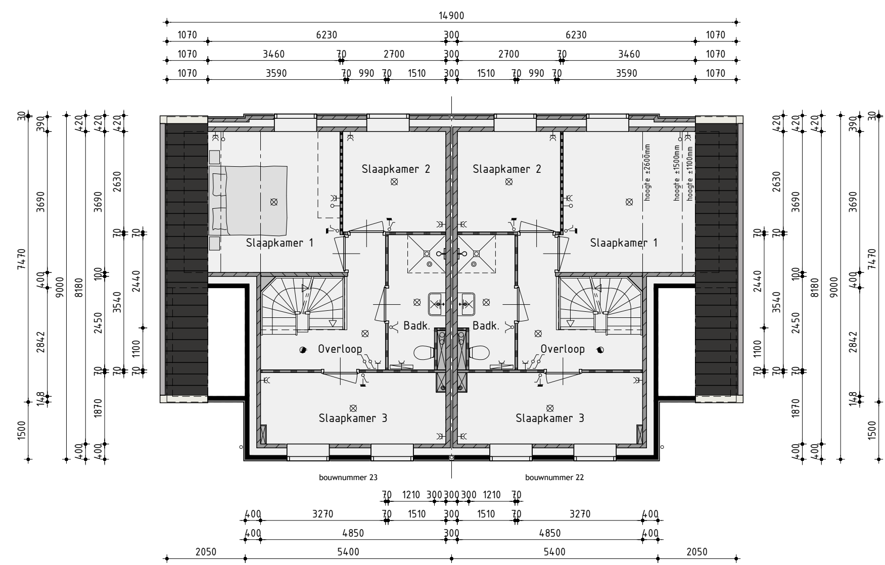
1ste Verdieping
