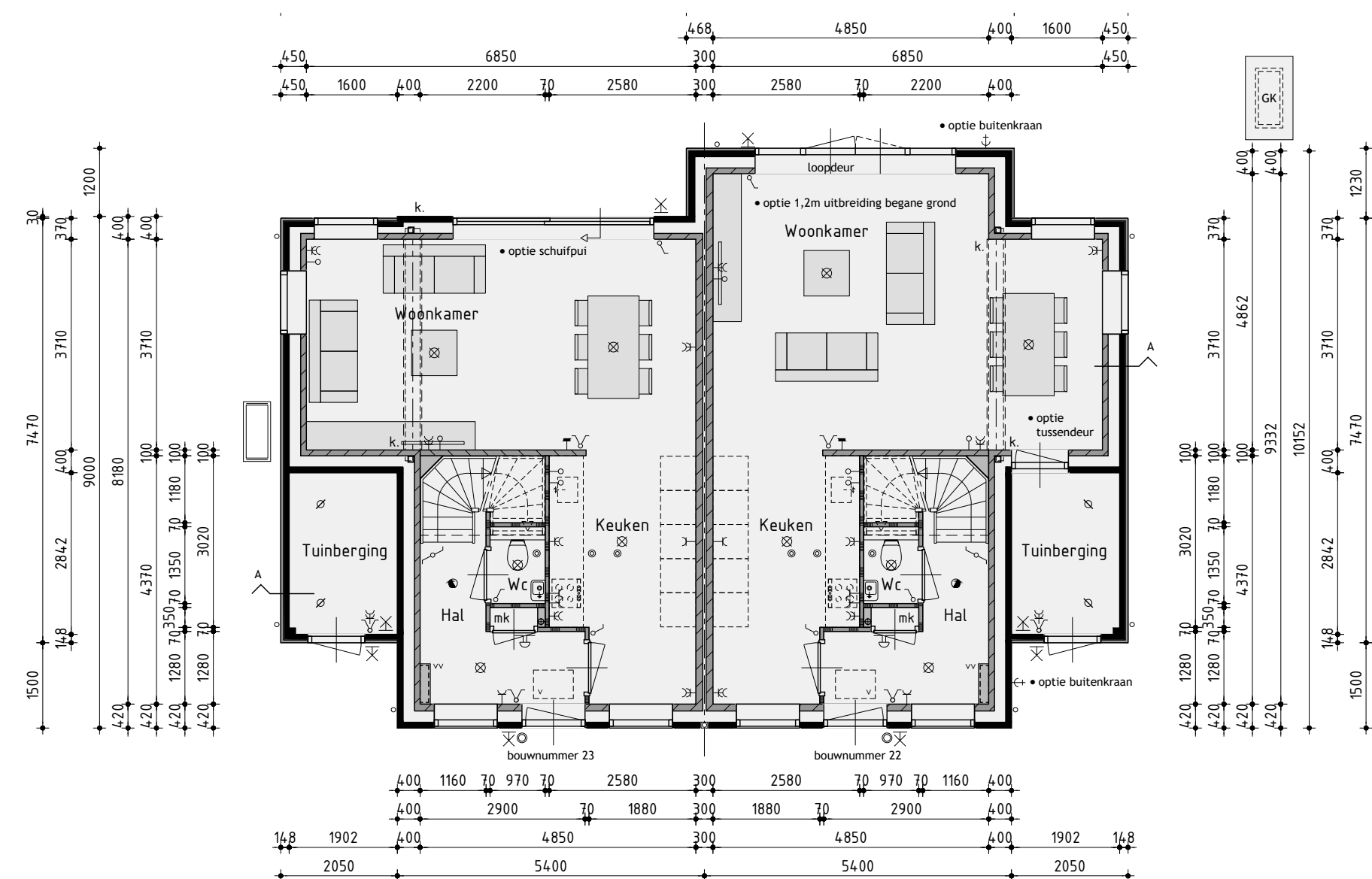
Begane grond
